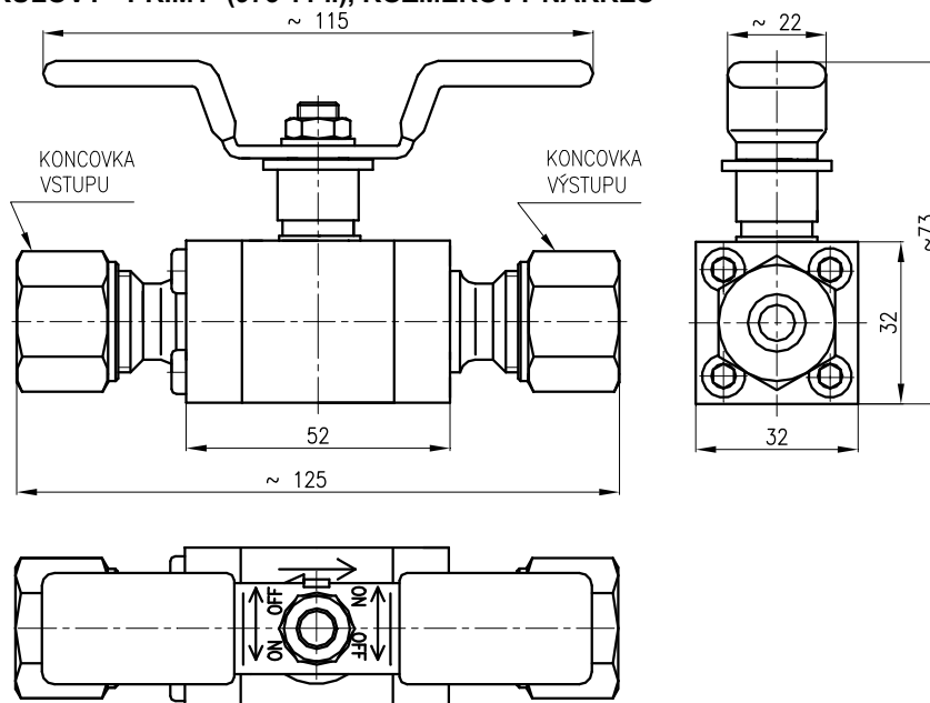
OBŘÁZEK 1 - KOHOUT KULOVÝ - PŘÍMÝ (973 11 ..), ROZMĚROVÝ NÁKRES
