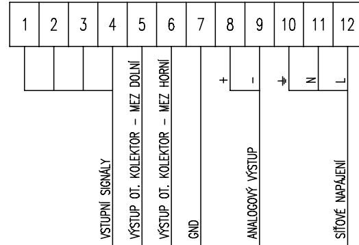
Se signalizací mezí a s analogovým výstupem
