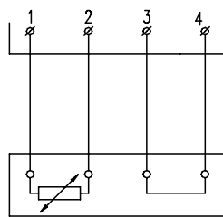
Odporové signály - čtyřvodič Snímač - v zapojení se smyčkou
