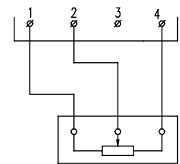
Odporový vysílač - třívodič
