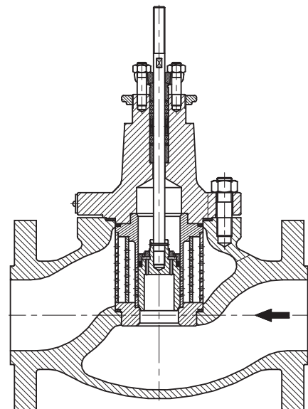
Obr. 1a Ventil BR12B s odlehčenou kuželkou
