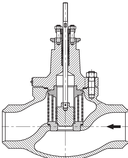
Obr. 1a Ventil BR12B s neodlehčenou kuželkou
