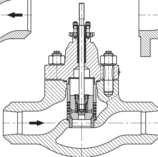
Obr. 1a Ventil BR12B s kuželkou odlehčenou pilotem
