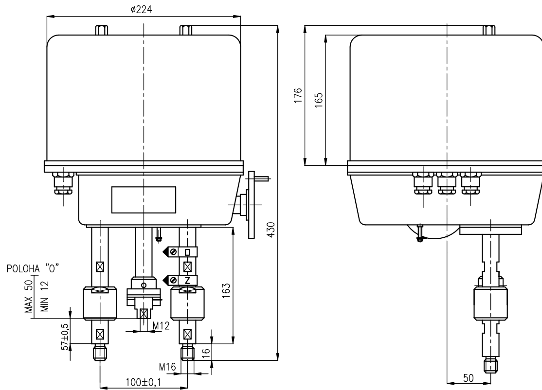
OBRAZEK 2 - ROZMĚROVÝ NÁKRES – PŘIPOJENÍ P3
